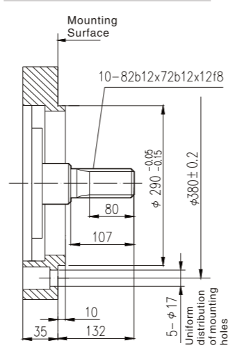
NHM16-** N
