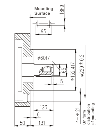
NHM16-** B 6
