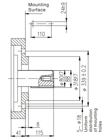
NHM16-** B 17
