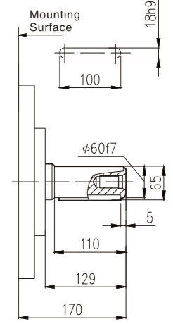
NHM16-** B 19
