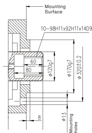
NHM16-** I 42
